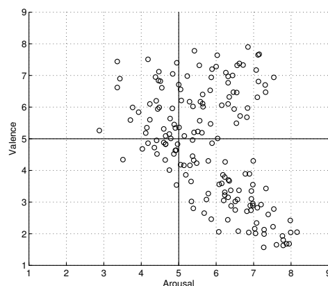
Fig. 1: Scatter plot of the IADS AV annotations
